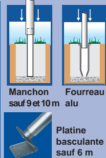
Platine basculante
